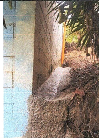
Foto 4: Mejoramiento de la cuneta de concreto.
